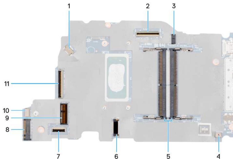
Rysunek 66. Złącza na płycie głównej
