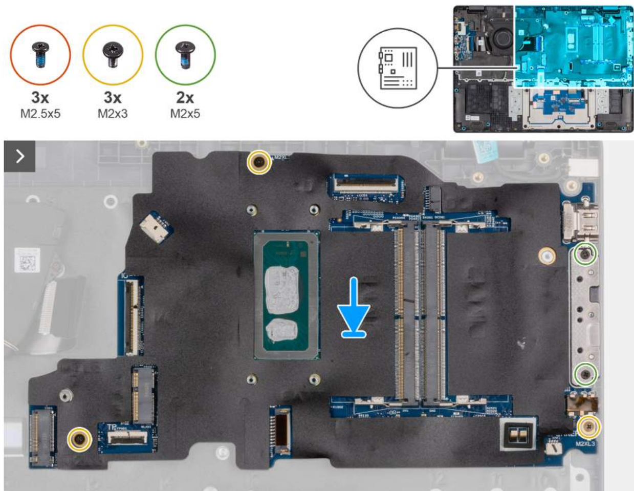
Rysunek 61. Instalowanie płyty głównej
