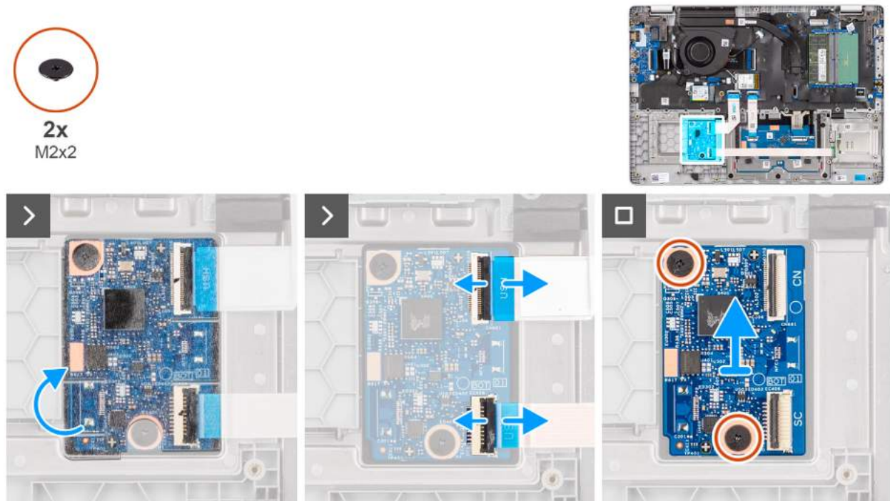
Rysunek 37. Wymontowywanie karty USH
