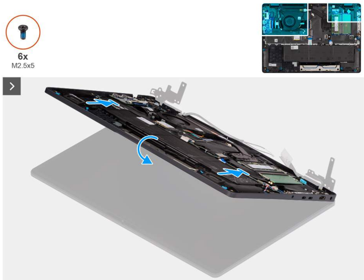
Rysunek 96. Instalowanie zestawu wyświetlacza
