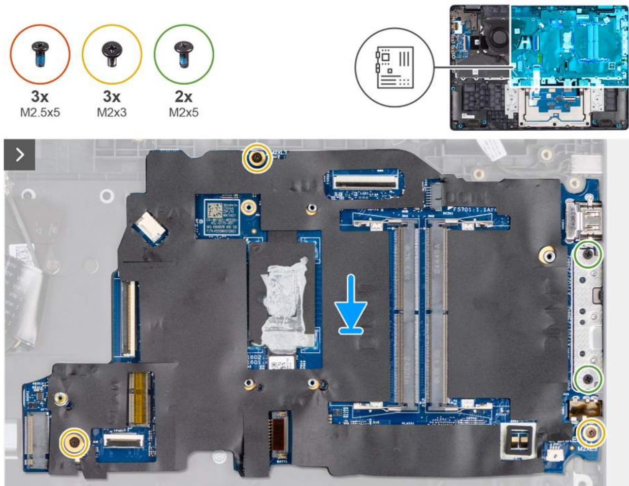
Rysunek 46. Instalowanie płyty głównej
