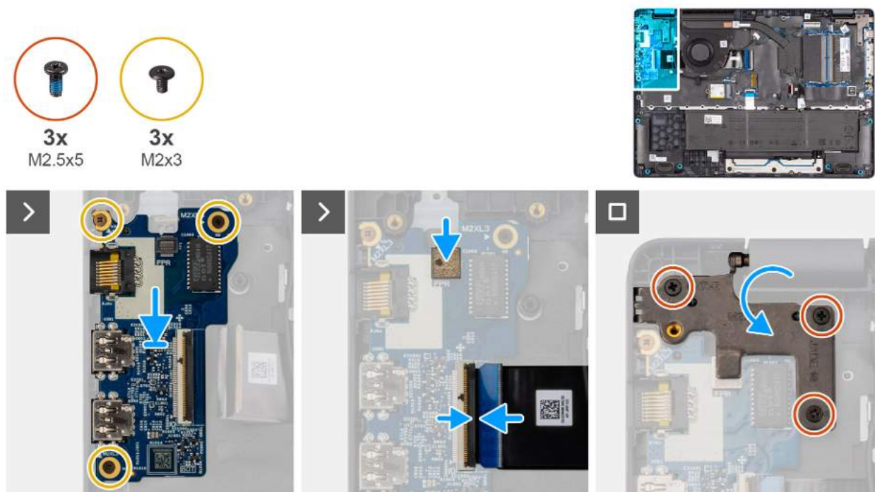
Rysunek 37. Instalowanie płyty we/wy
