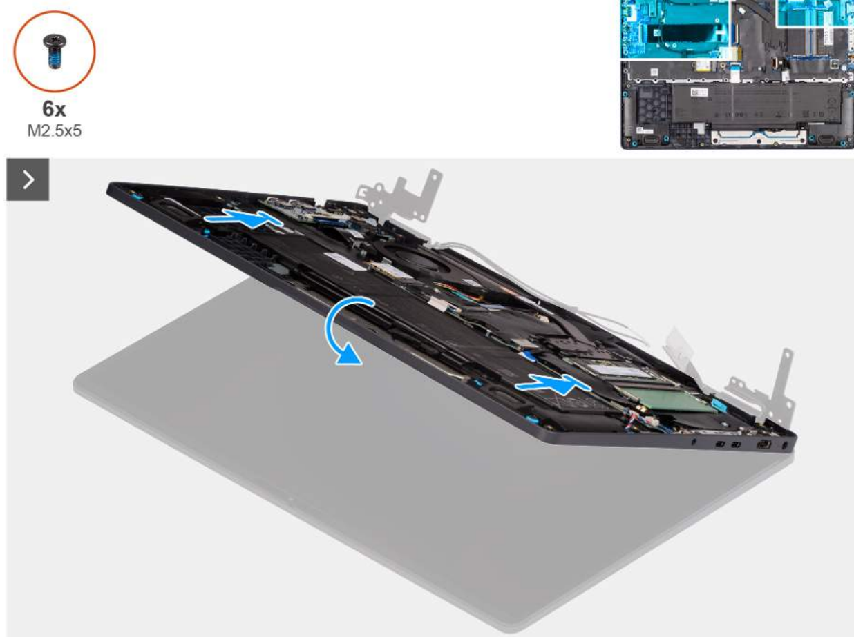
Rysunek 65. Instalowanie zestawu wyświetlacza
