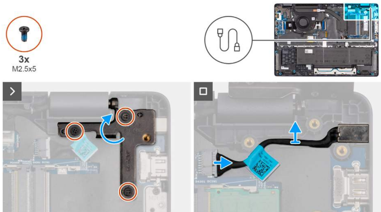
Rysunek 32. Wymontowywanie gniazda zasilacza
