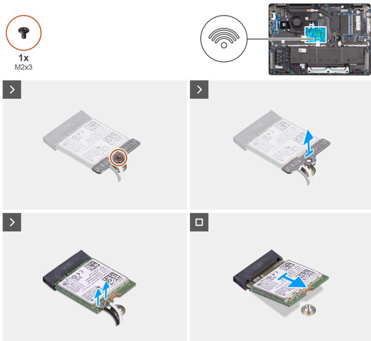
Rysunek 25. Wymontowywanie karty sieci bezprzewodowej
