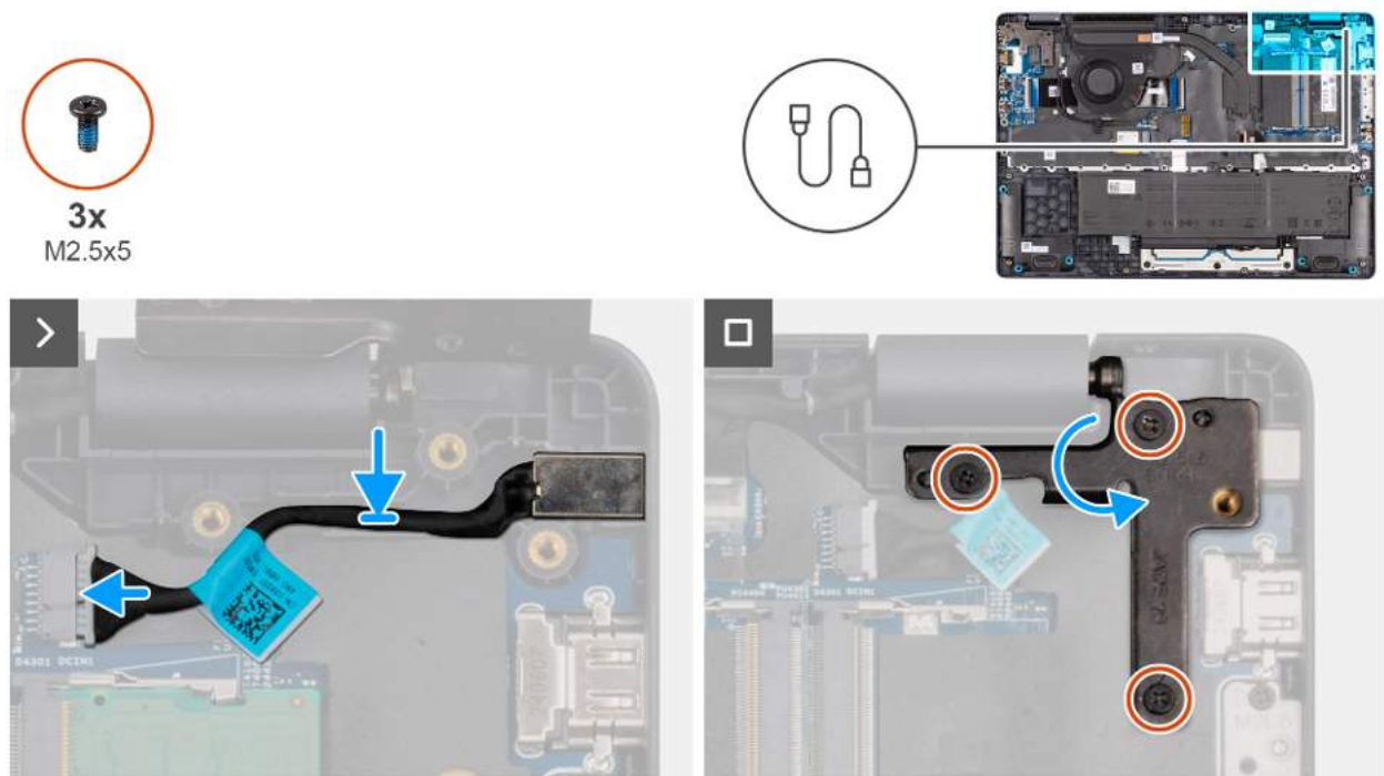
Rysunek 33. Instalowanie gniazda zasilacza
