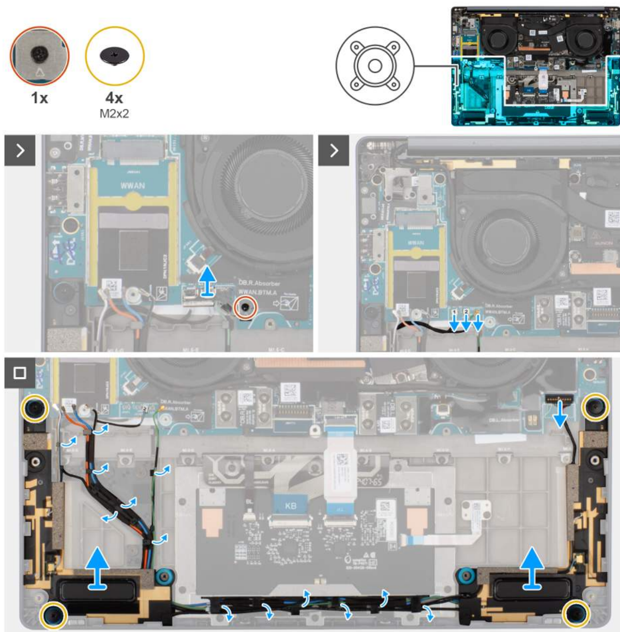
Rysunek 36. Wyjmowanie głośników z antenami (konfiguracja WWAN)
