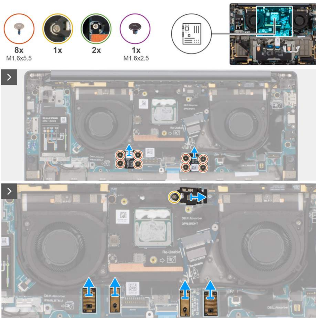
Rysunek 64. Wymontowywanie płyty głównej
