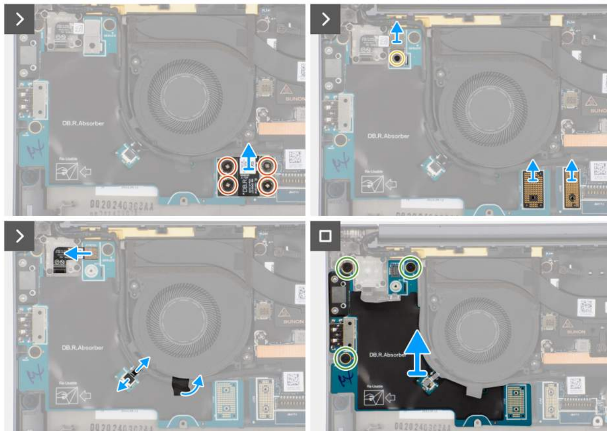
Rysunek 44. Wyjmowanie prawej płyty we/wy (bez anten WWAN)
