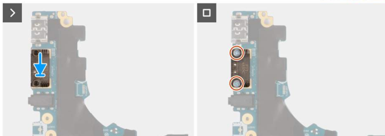
Rysunek 55. Instalowanie odpowiedniego modułu USB typu C
