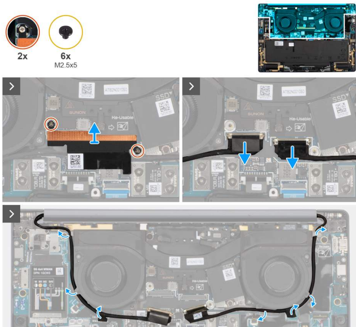
Rysunek 58. Odłącz kable wyświetlacza i kamery
