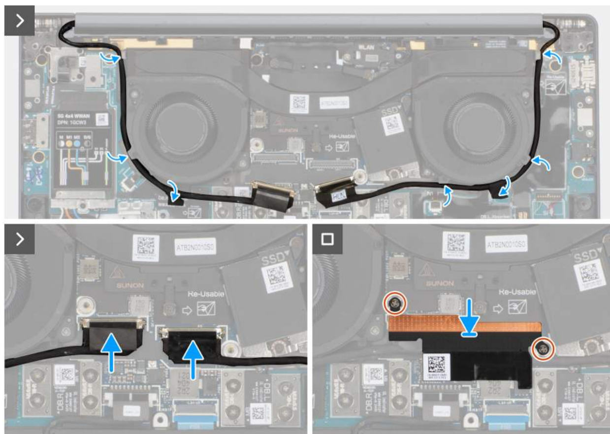
Rysunek 62. Podłączanie przewodów wyświetlacza i kamery
