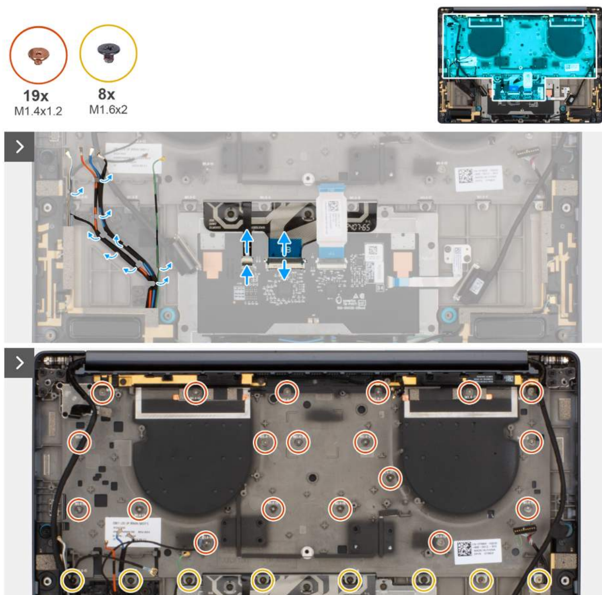
Rysunek 73. Wymontowywanie zestawu klawiatury
