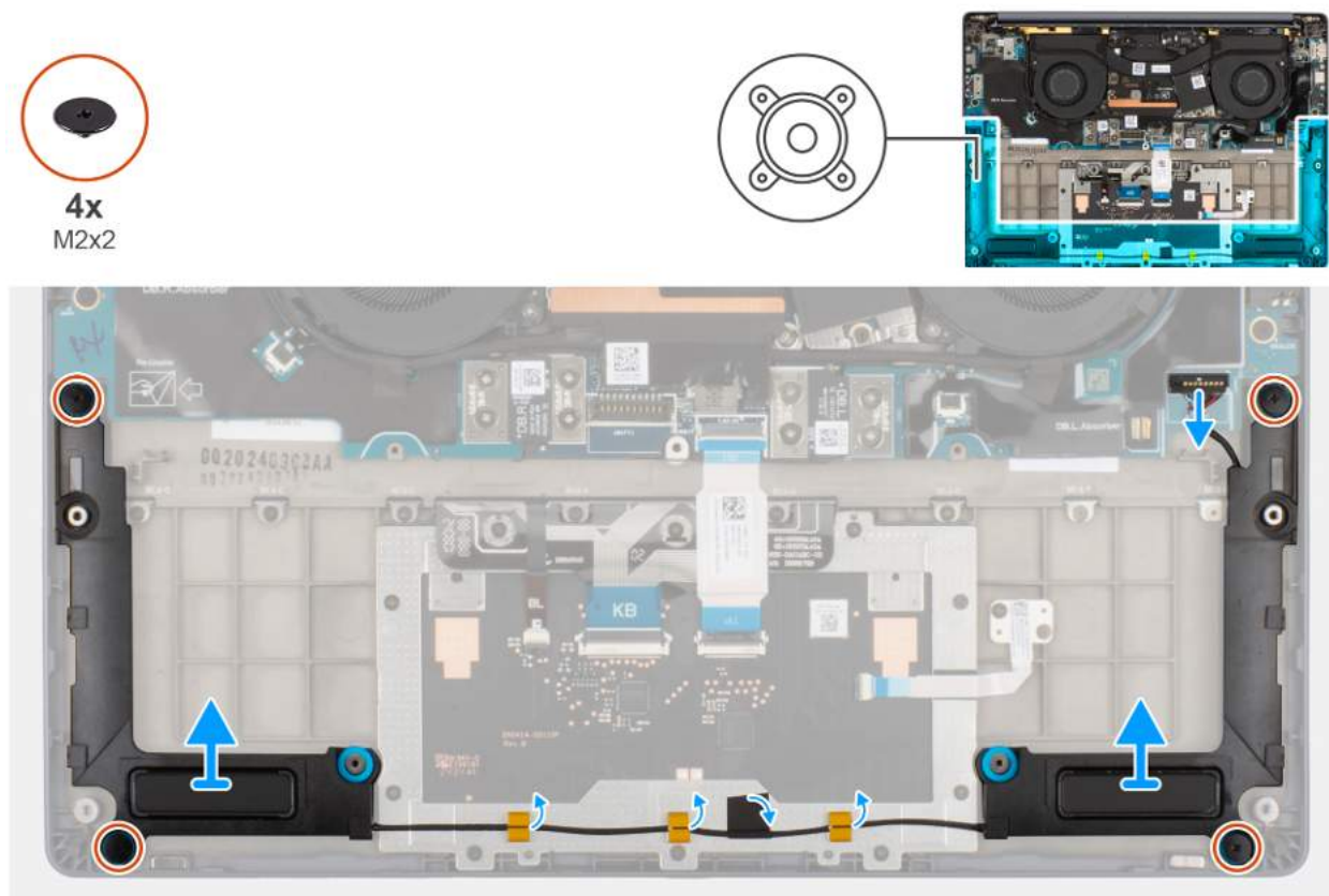
Rysunek 34. Wyjmowanie głośników bez anteny (konfiguracja WLAN)
