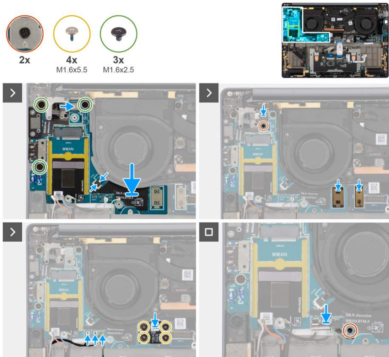
Rysunek 50. Instalowanie prawej płyty we/wy (z WWAN)
