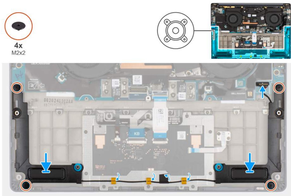
Rysunek 35. Instalowanie głośników (bez WWAN)
