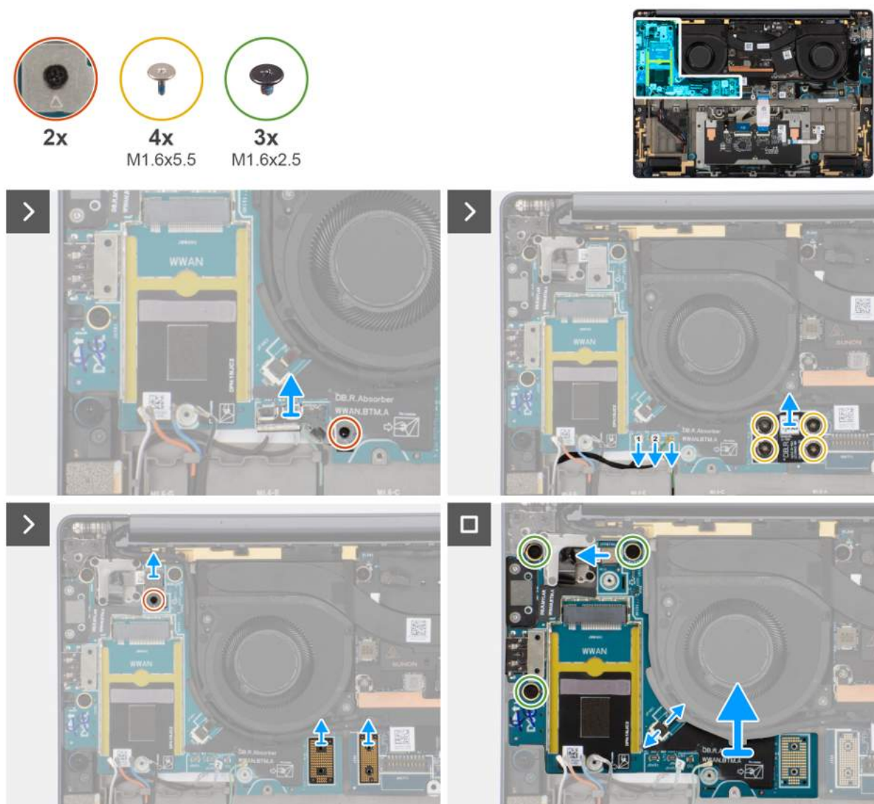
Rysunek 48. Wyjmowanie prawej płyty we/wy (z WWAN)
