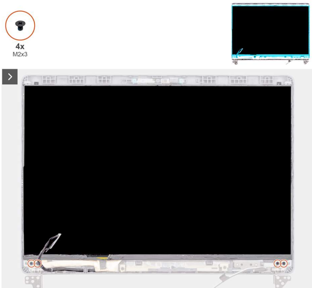
Rysunek 60. Wymontowywanie wyświetlacza
