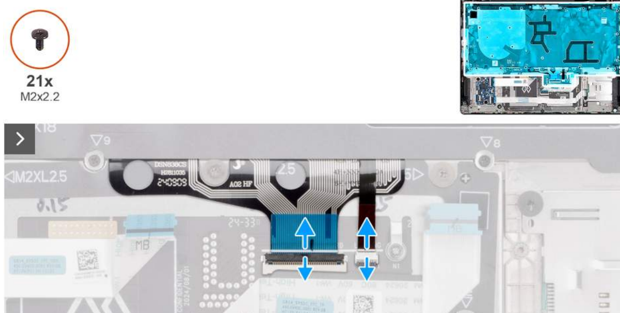
Rysunek 94. Wymontowywanie klawiatury
