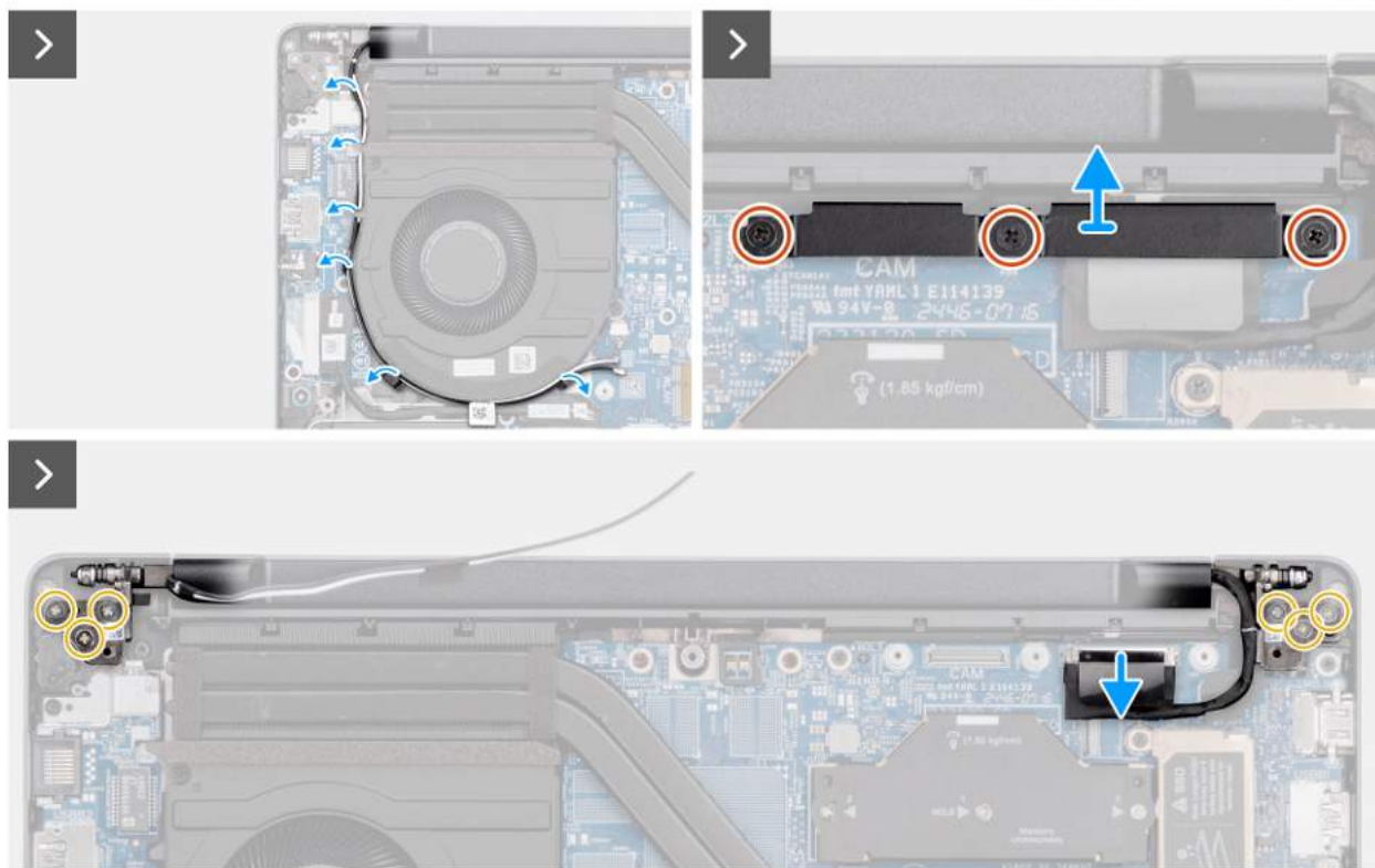
Rysunek 47. Wymontowywanie zestawu wyświetlacza
