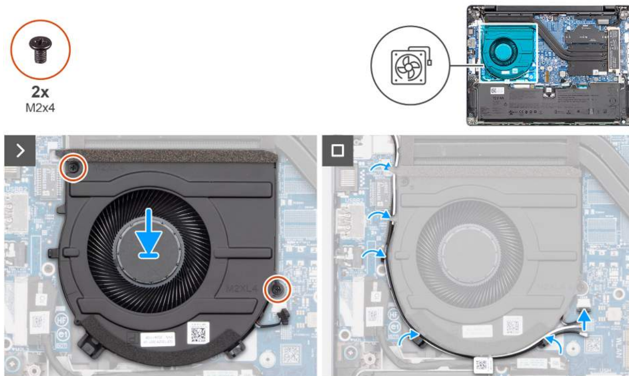
Rysunek 32. Instalowanie wentylatora
