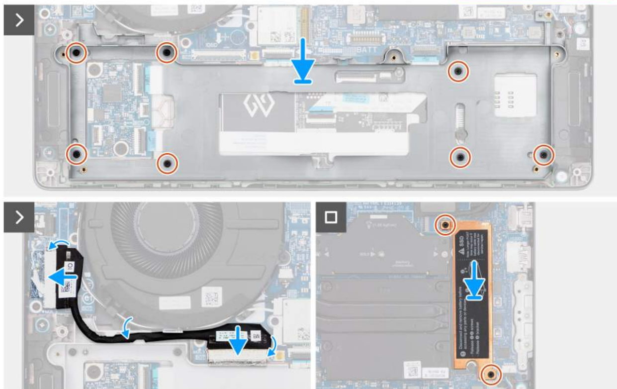
Rysunek 34. Instalowanie ramy baterii
