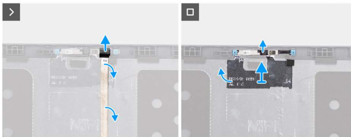
Rysunek 70. Wymontowywanie kamery
