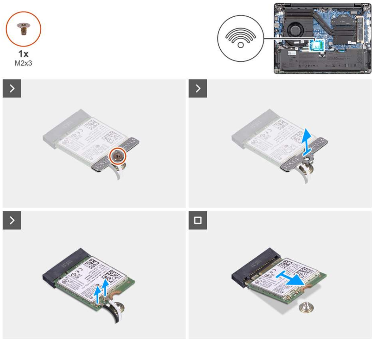
Rysunek 26. Wymontowywanie karty sieci bezprzewodowej
