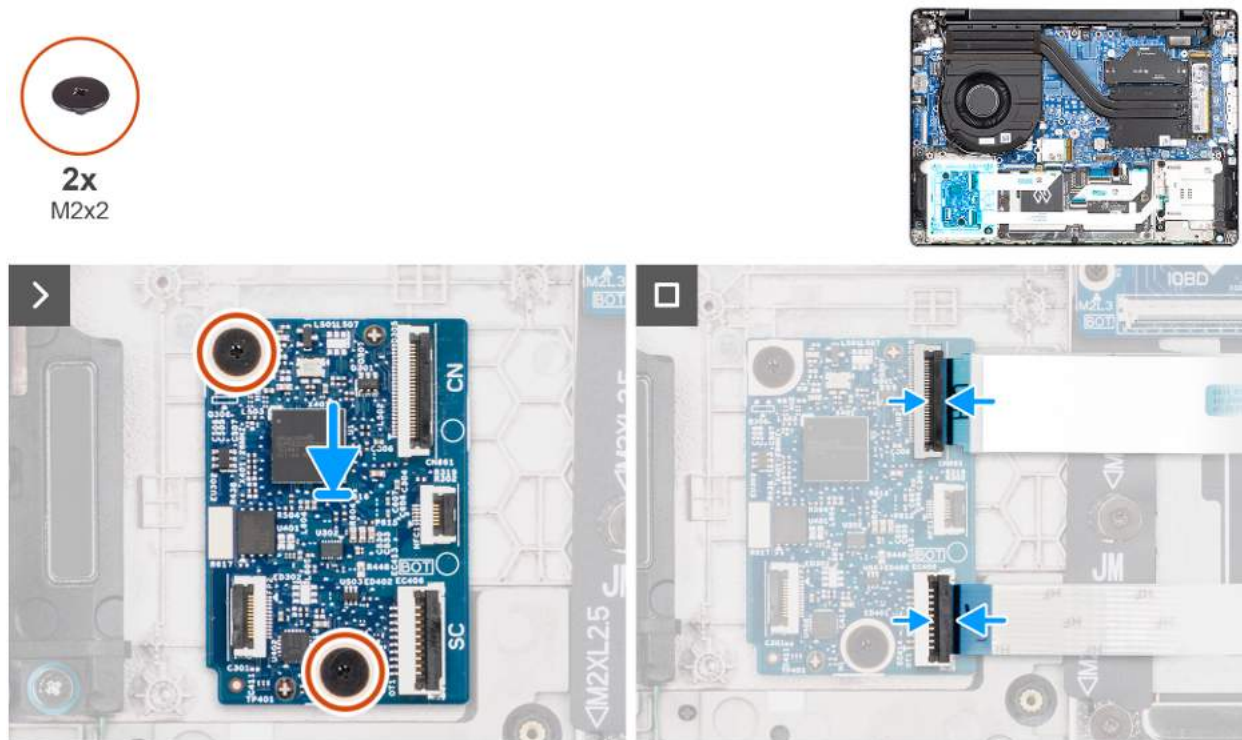
Rysunek 36. Instalowanie karty USH
