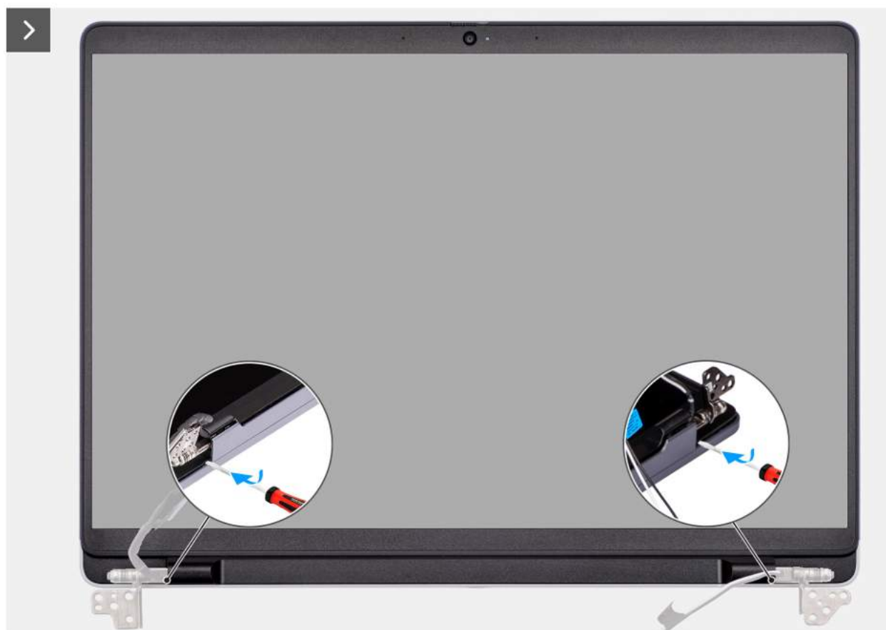
Rysunek 52. Wymontowywanie ramki wyświetlacza
