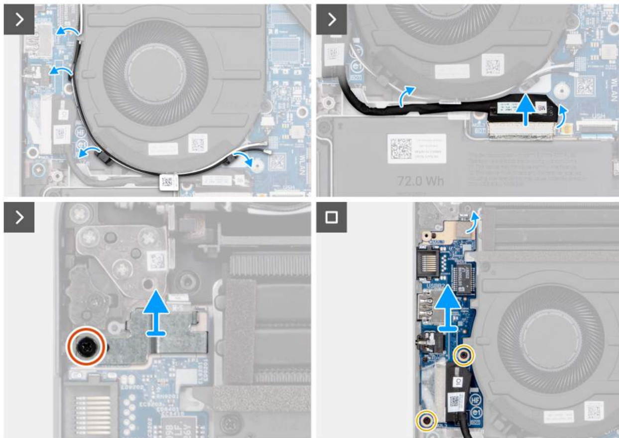
Rysunek 43. Wymontowywanie płyty we/wy
