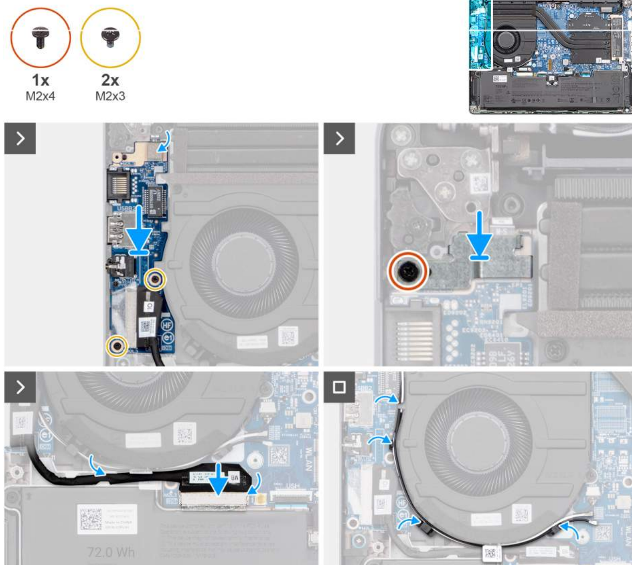
Rysunek 44. Instalowanie płyty we/wy
