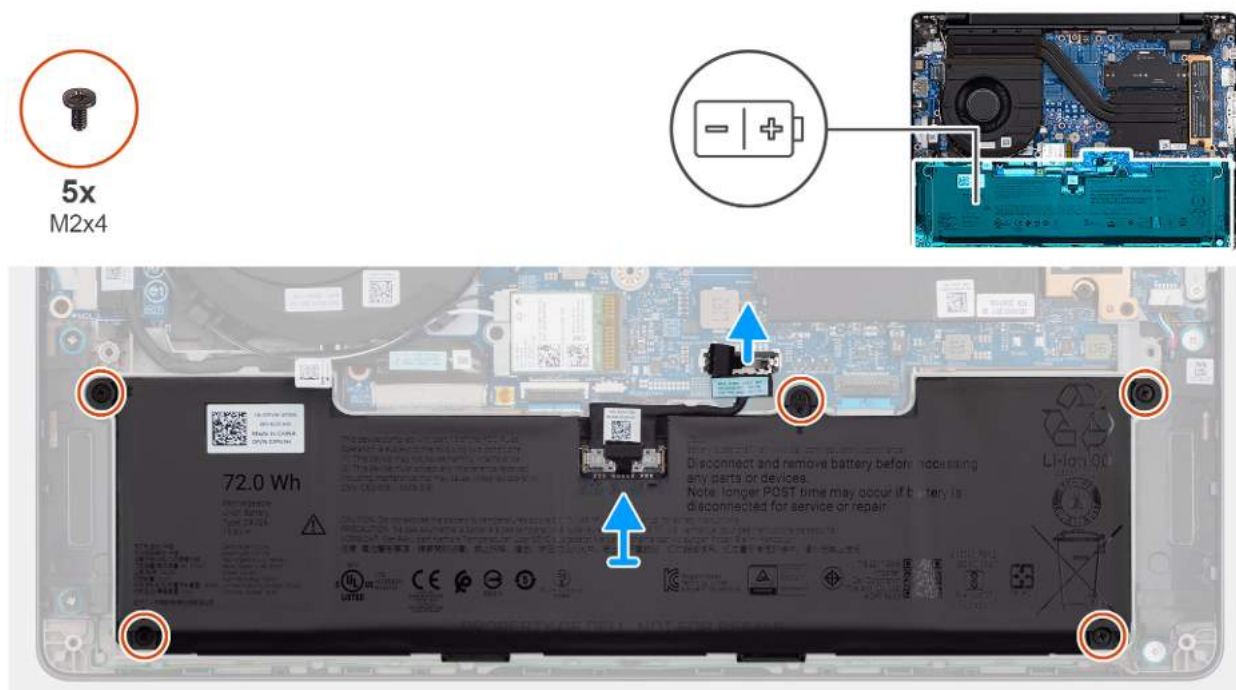
Rysunek 16. Wymontowywanie baterii
