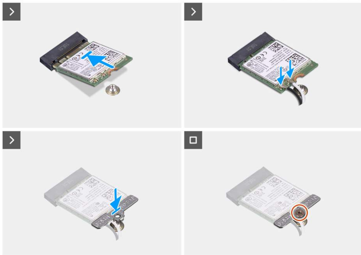
Rysunek 27. Instalowanie karty sieci bezprzewodowej
