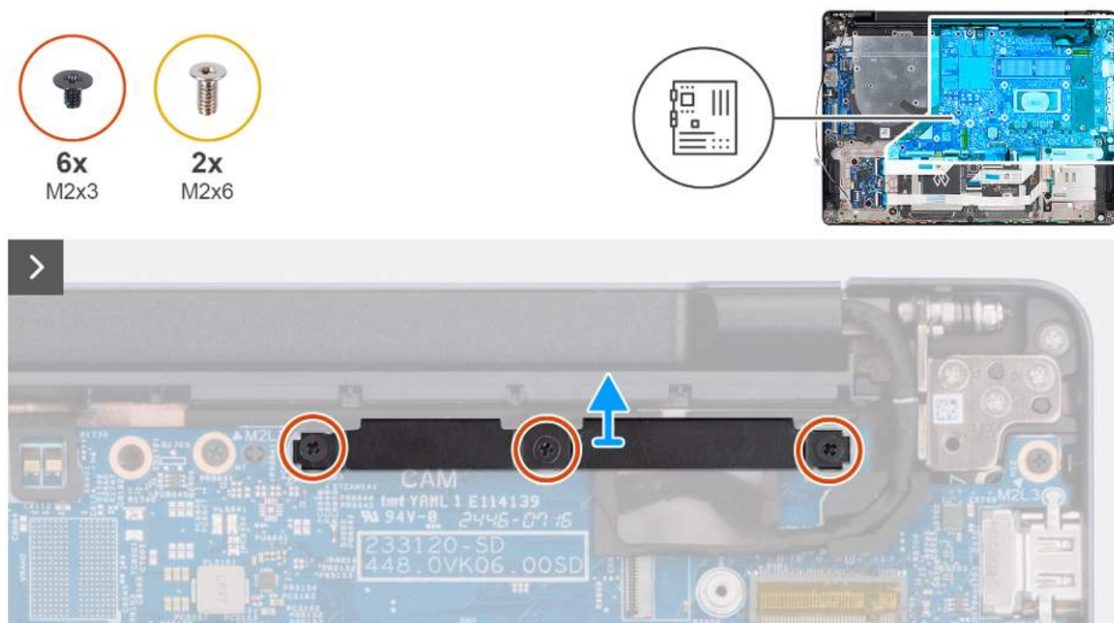
Rysunek 75. Wymontowywanie płyty głównej
