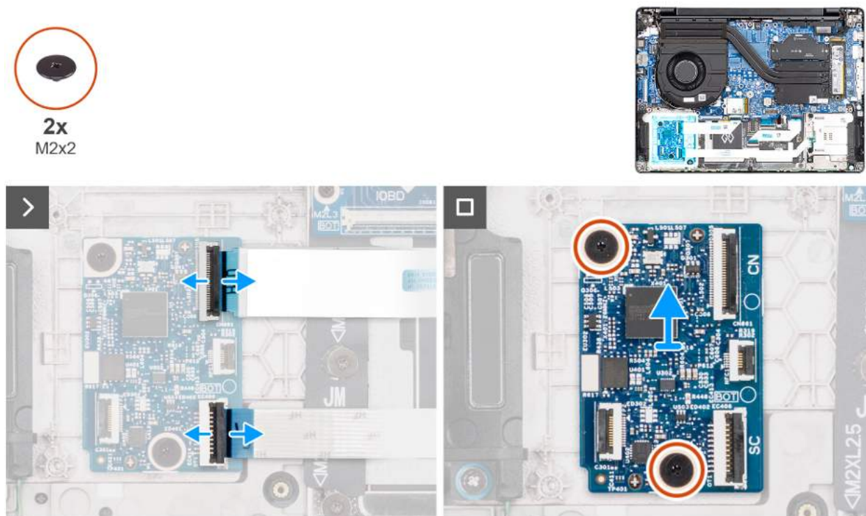
Rysunek 35. Wymontowywanie karty USH
