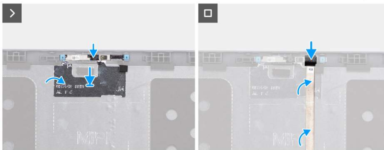
Rysunek 71. Instalowanie kamery
